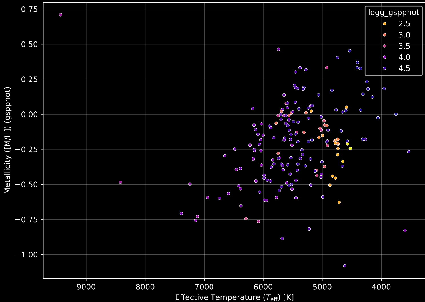
APOGEE DR17 Field: [186+48] Stellar Population Parameters (n= 190)
